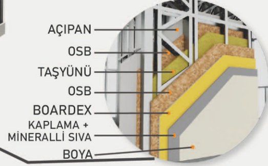
DIŞ DUVAR KAPLAMA DETAYI
