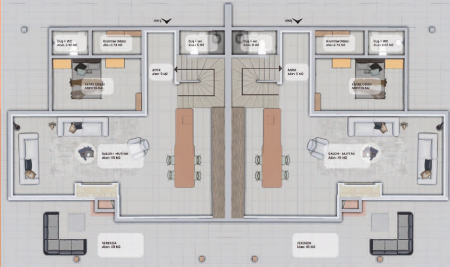
Zemin Kat Planı
