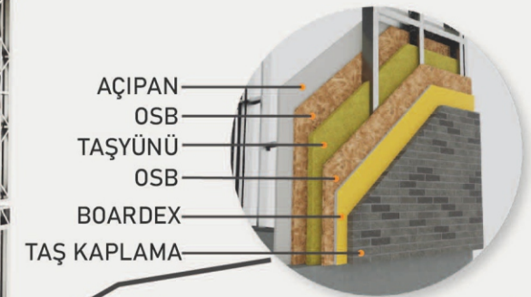
TAŞ KAPLAMA DETAYI
