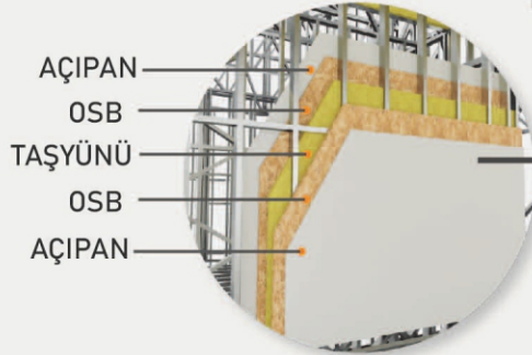
İÇ DUVAR KAPLAMA DETAYI
